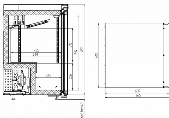
DP102-S с осевым вентилятором
