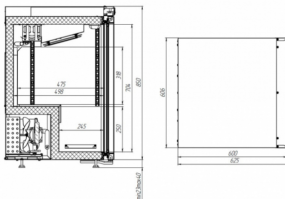
DP102-S с осевым вентилятором
