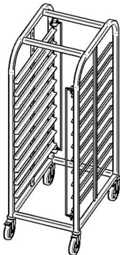
Рис.11 ТШГ-10-1/1
