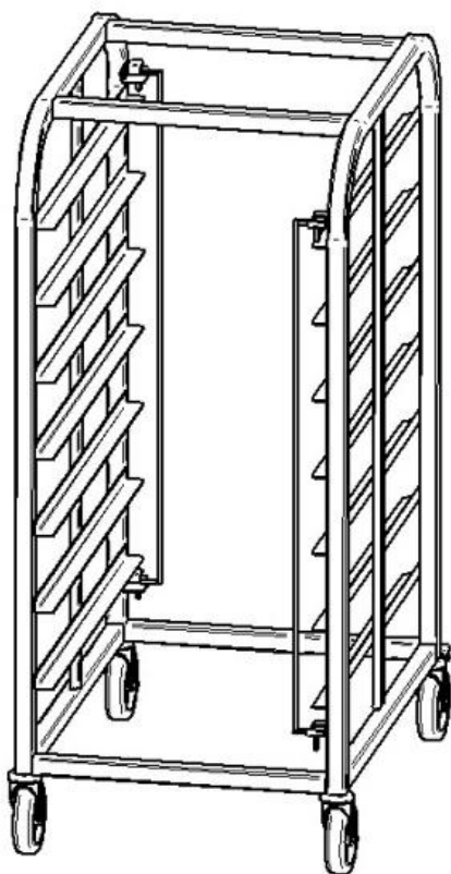
Рис.1 ТШГ-7-6-4
