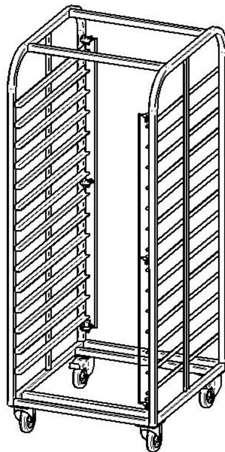
Рис.10 ТШГ-14-2/1М
