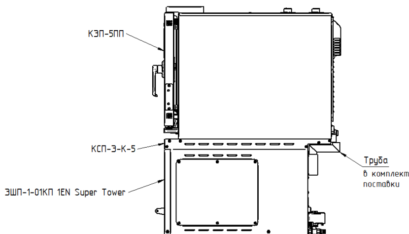
Рис.2 Общий вид "колонны" в сборе.
